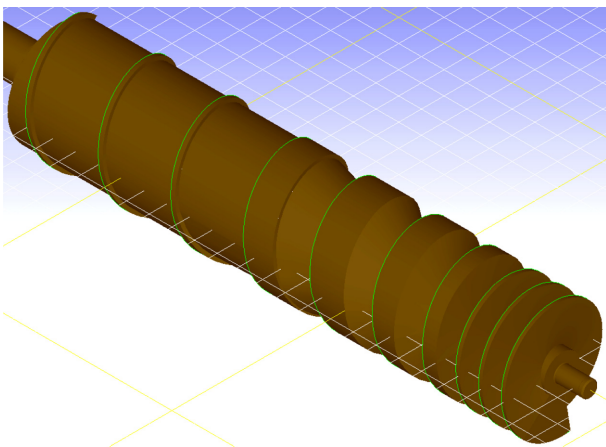
Fig. 6 Edge selection
