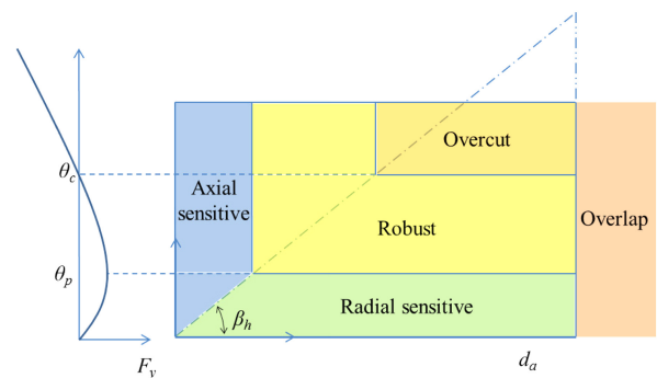
(d) Property zones of up milling
